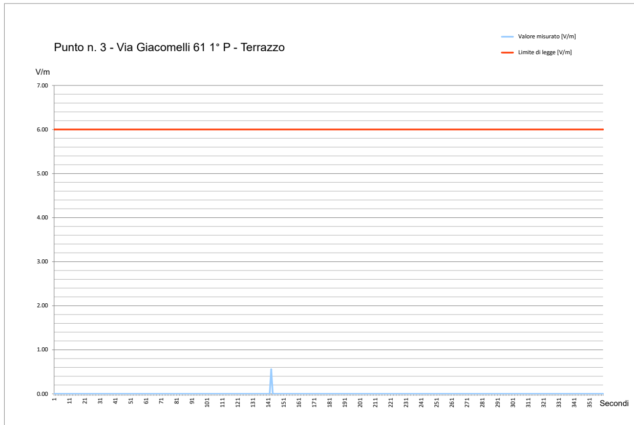
Fig. 15 Grafico Misura di Campo Elettromagnetico a RadioFrequenza – Punto #3
