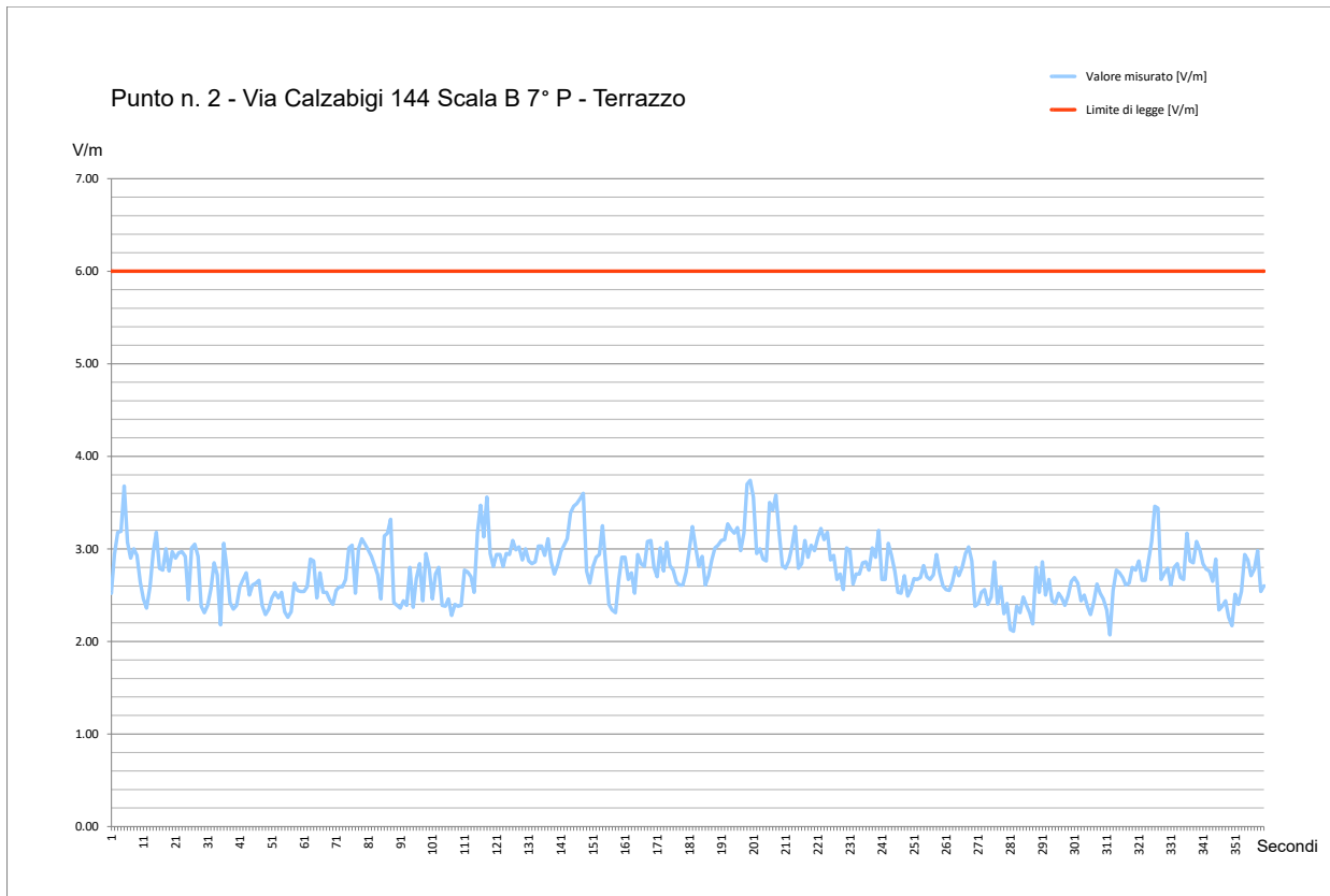
Fig. 12 Grafico Misura di Campo Elettromagnetico a RadioFrequenza – Punto #2
