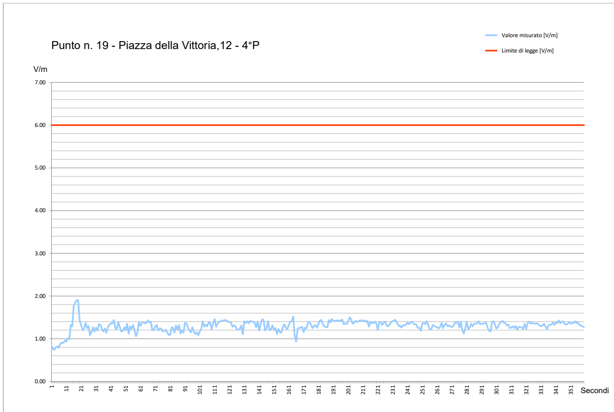
Fig. 63 Grafico Misura di Campo Elettromagnetico a RadioFrequenza – Punto #19
