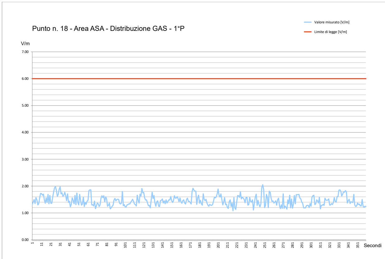
Fig. 60 Grafico Misura di Campo Elettromagnetico a RadioFrequenza – Punto #18
