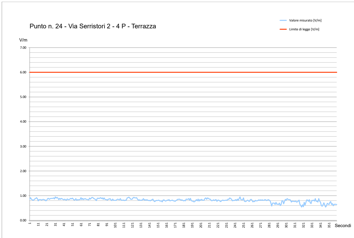
Fig. 78 Grafico Misura di Campo Elettromagnetico a RadioFrequenza – Punto #24
