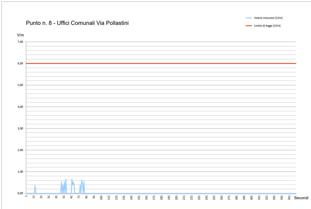
Fig. 30 Grafico Misura di Campo Elettromagnetico a RadioFrequenza – Punto #8
