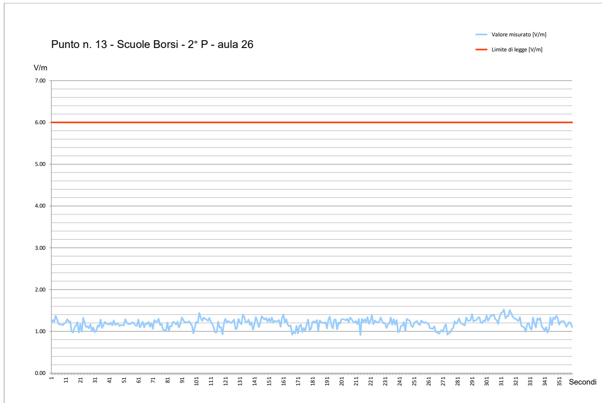
Fig. 45 Grafico Misura di Campo Elettromagnetico a RadioFrequenza – Punto #13
