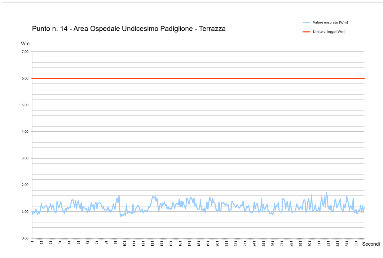
Fig. 48 Grafico Misura di Campo Elettromagnetico a RadioFrequenza – Punto #14
