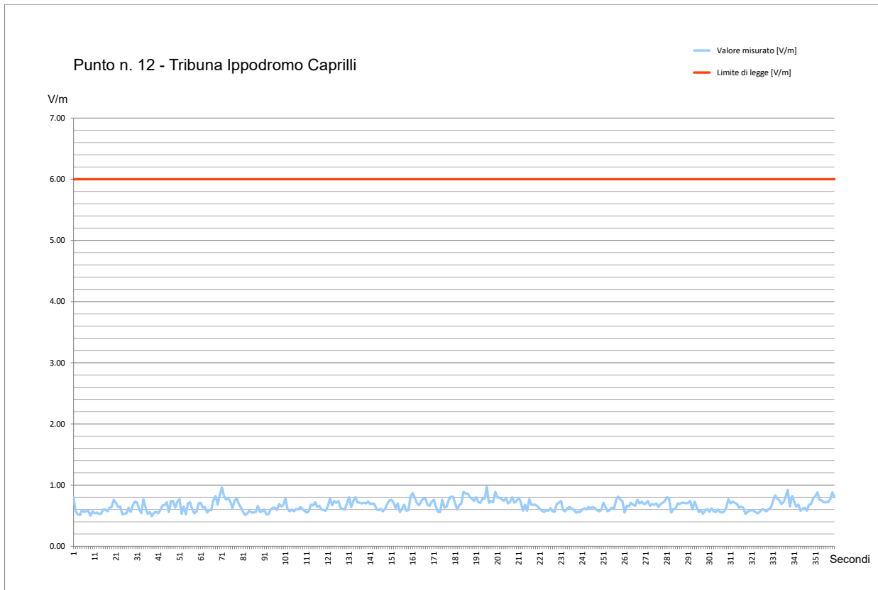
Fig. 42 Grafico Misura di Campo Elettromagnetico a RadioFrequenza – Punto #12
