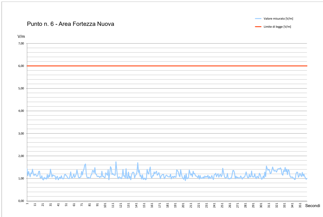
Fig. 24 Grafico Misura di Campo Elettromagnetico a RadioFrequenza – Punto #6
