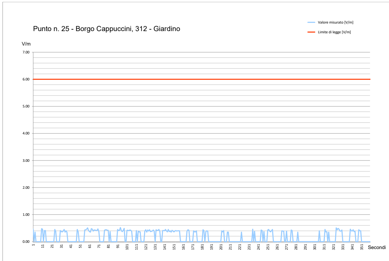
Fig. 81 Grafico Misura di Campo Elettromagnetico a RadioFrequenza – Punto #25
