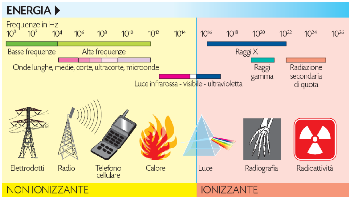
Fig. 1 Spettro Elettromagnetico
