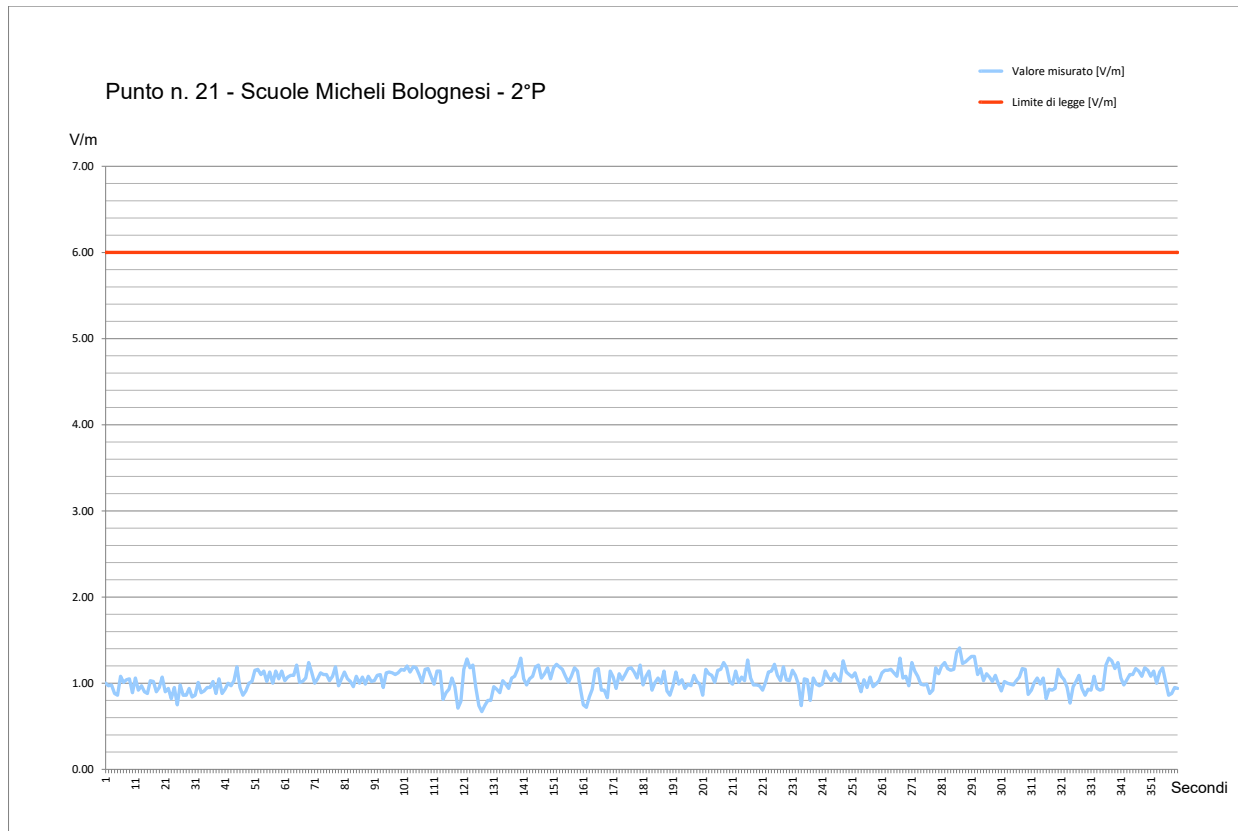
Fig. 69 Grafico Misura di Campo Elettromagnetico a RadioFrequenza – Punto #21
