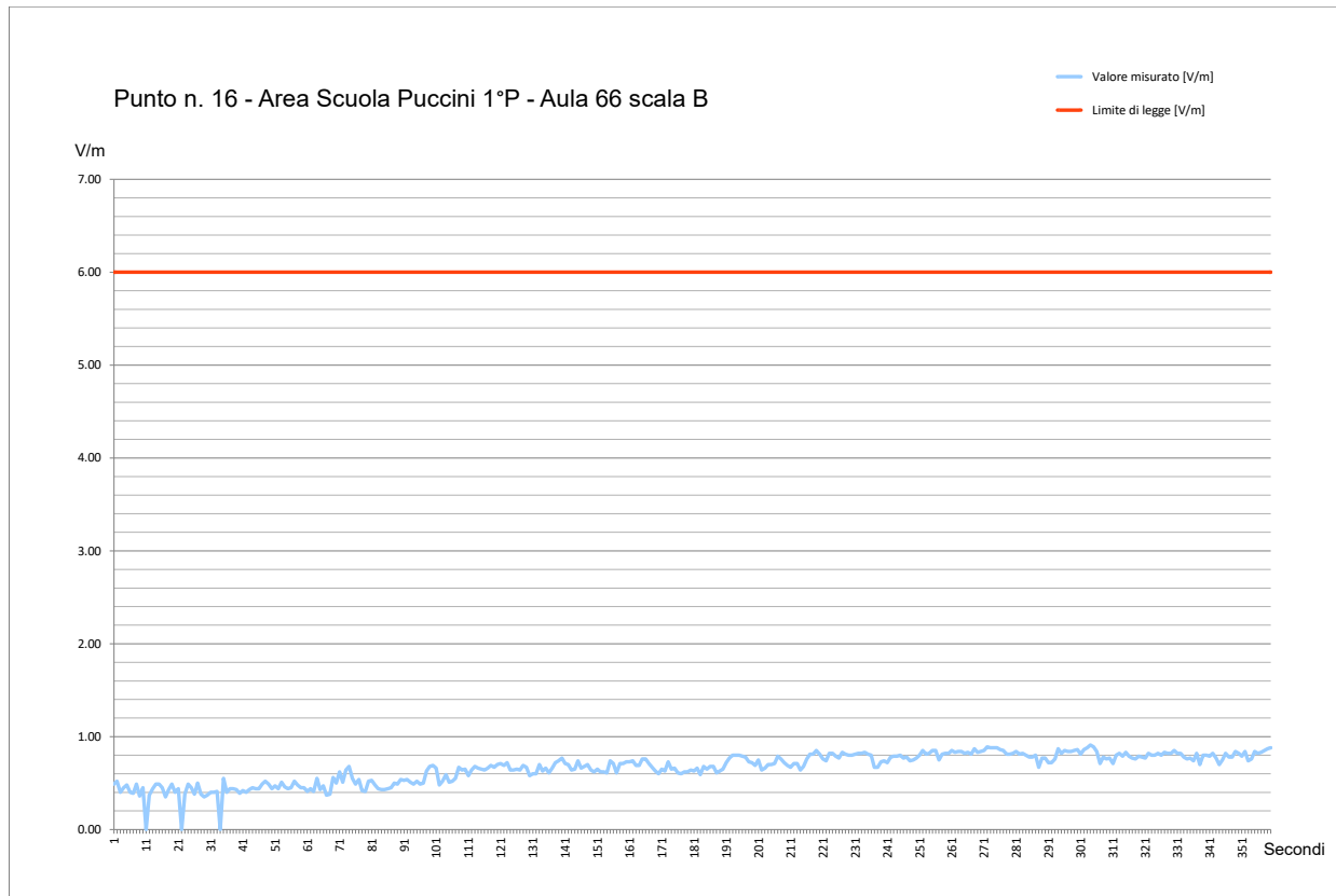
Fig. 54 Grafico Misura di Campo Elettromagnetico a RadioFrequenza – Punto #16
