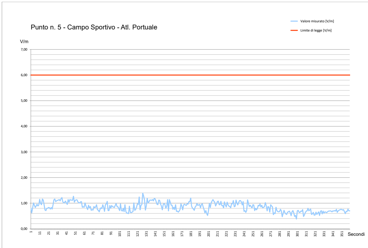
Fig. 21 Grafico Misura di Campo Elettromagnetico a RadioFrequenza – Punto #5
