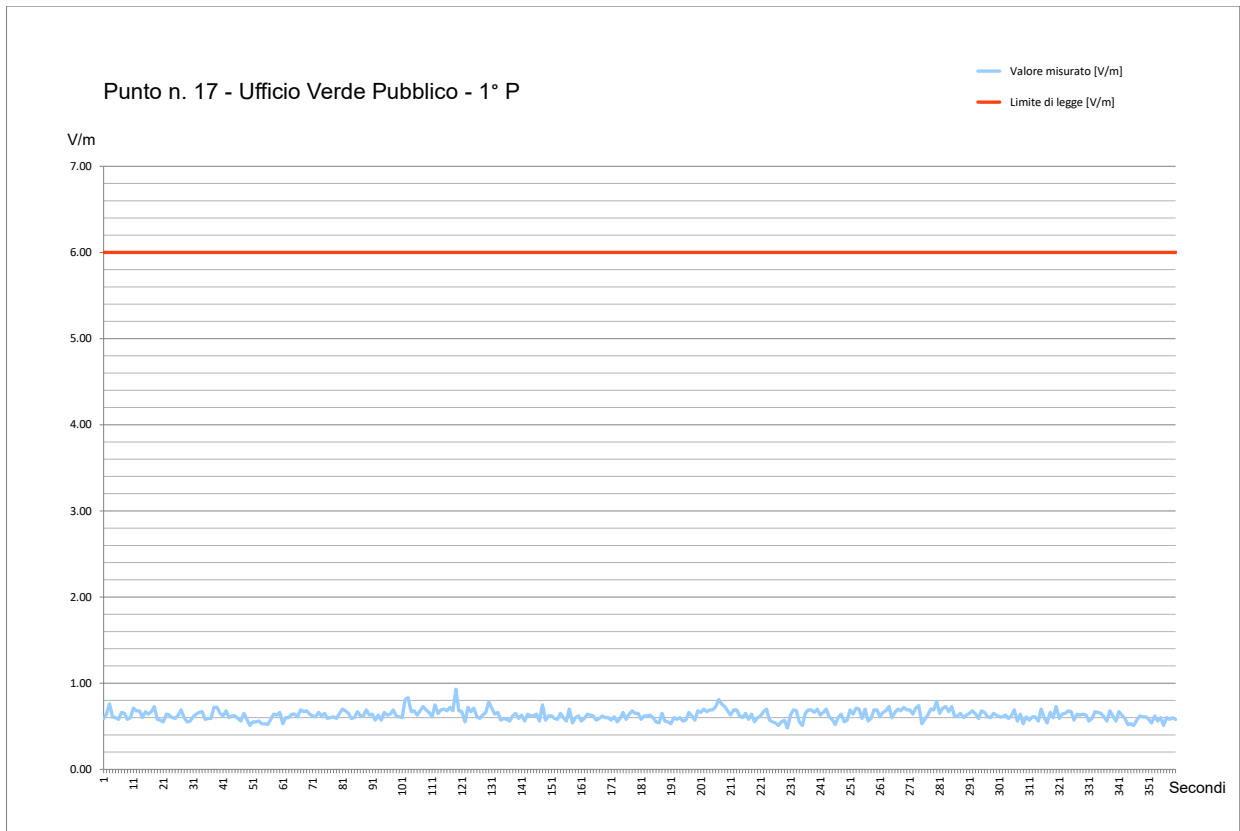
Fig. 57 Grafico Misura di Campo Elettromagnetico a RadioFrequenza – Punto #17
