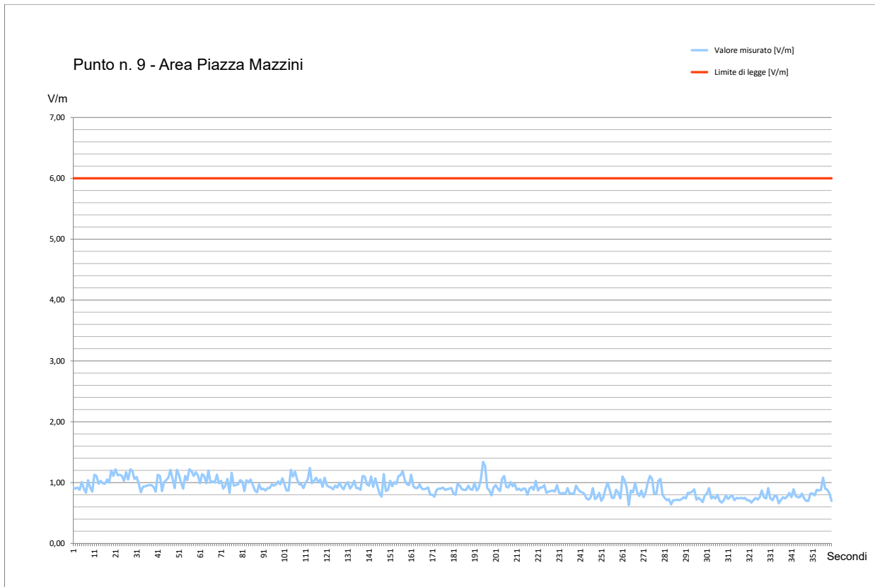
Fig. 33 Grafico Misura di Campo Elettromagnetico a RadioFrequenza – Punto #9
