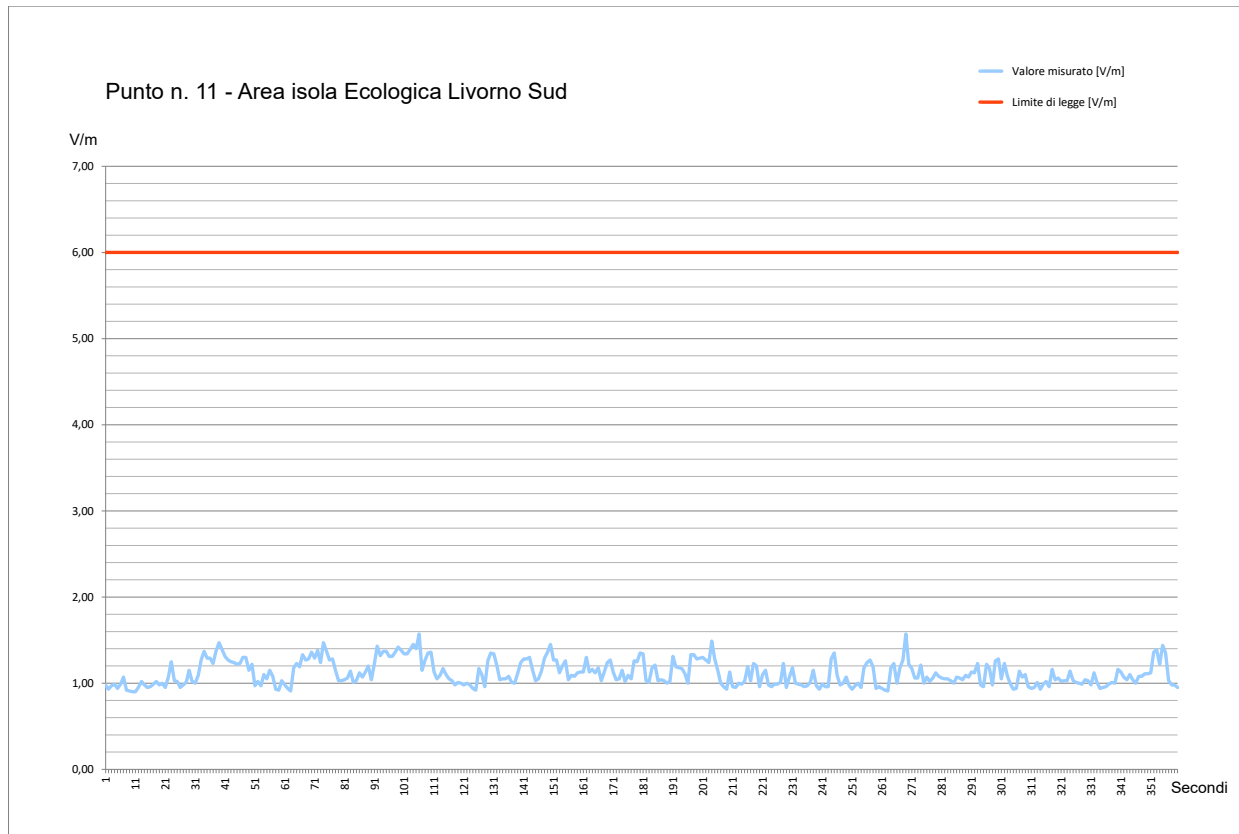
Fig. 39 Grafico Misura di Campo Elettromagnetico a RadioFrequenza – Punto #11
