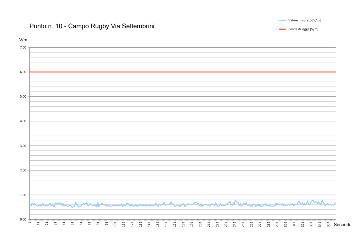
Fig. 36 Grafico Misura di Campo Elettromagnetico a RadioFrequenza – Punto #10
