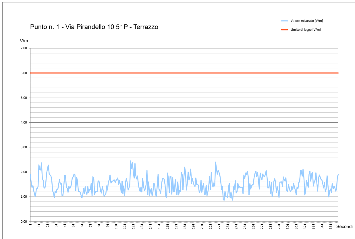
Fig. 9 Grafico Misura di Campo Elettromagnetico a RadioFrequenza – Punto #1
