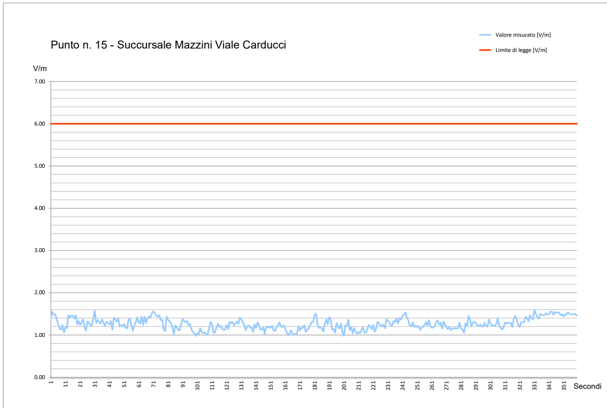
Fig. 51 Grafico Misura di Campo Elettromagnetico a RadioFrequenza – Punto #15
