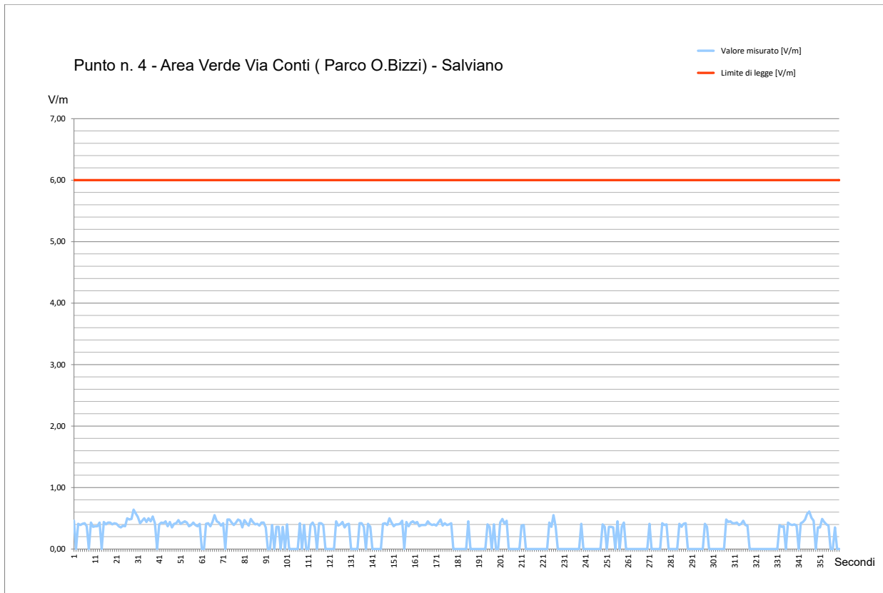
Fig. 18 Grafico Misura di Campo Elettromagnetico a RadioFrequenza – Punto #4
