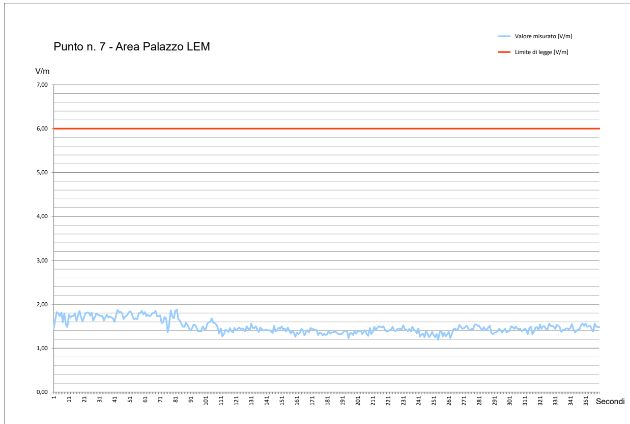
Fig. 27 Grafico Misura di Campo Elettromagnetico a RadioFrequenza – Punto #7
