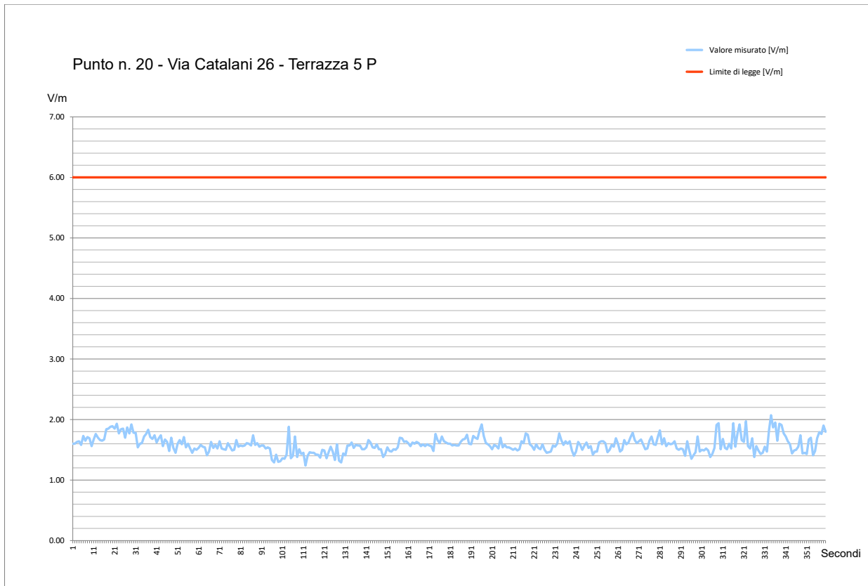
Fig. 66 Grafico Misura di Campo Elettromagnetico a RadioFrequenza – Punto #20
