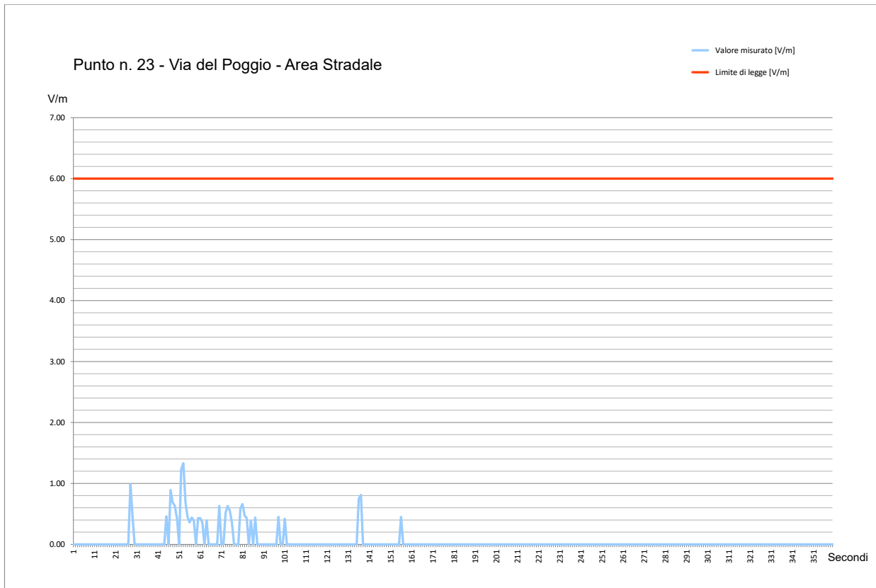
Fig. 75 Grafico Misura di Campo Elettromagnetico a RadioFrequenza – Punto #23
